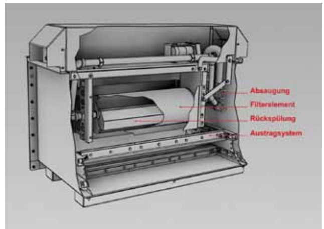
Funktionsweise eines Unterdrucksaugfilters
